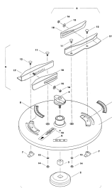
ETB-007803, Tarcze do rozsiewu granicznego TS 15-18
