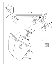
ETB-007805, Ekran rozsiewu granicznego
