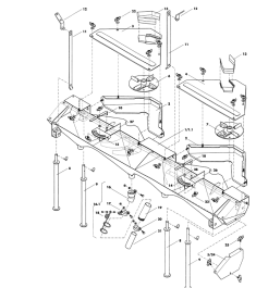
ETB-007826, Lejek środkowy do urządzenia rozsiewającego R4, R6, R8
