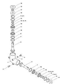
ETB-007807, Przekładnia kątowa
