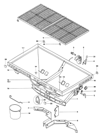
ETB-007795, Rama ze zbiornikiem
