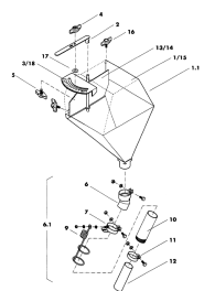
ETB-007827, Lejek zewnętrzny do urządzenia rozsiewającego R6
