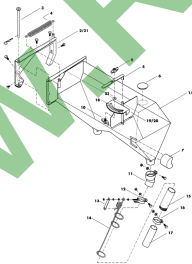
ETB-007828, Lejek odchylany do urządzenia rozsiewającego R8
