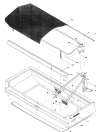
ETB-007820, Nadstawka nad zbiornik L3000
