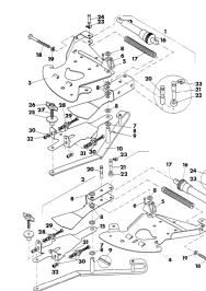
ETB-007814, System podwójnych zasuw z Amatron (2/2)
