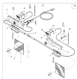
ETB-007823, Oświetlenie tylne
