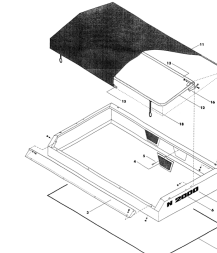
ETB-007818, Nadstawka nad zbiornik N i składana plandeka
