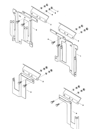
ETB-007824, Uchwyt oświetlenia do świateł nasadzanych i tablic ostrzegawczych postojowych
