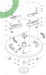
ETB-007801, Tarcze do rozsiewu granicznego TS 5-9
