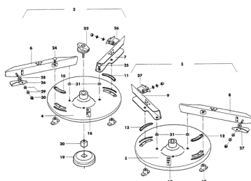
ETB-007799, Tarcze rozsiewające OS 20-28
