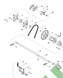
ETB-007809, Walek mieszadła i jarzmo napinające do łańcucha
