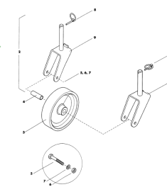
ETB-007822, Urządzenie transportowe i postojowe
