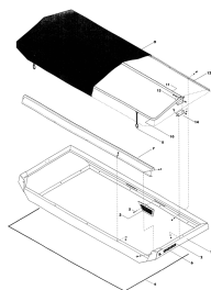
ETB-007819, Nadstawka nad zbiornik L i składana plandeka
