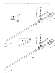
ETB-007815, Siłownik hydr. pojedynczej zasuw jednostronnego działania
