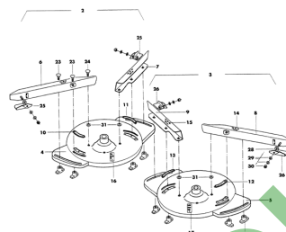
ETB-007800, Tarcze rozsiewające OS 30-36
