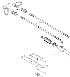
ETB-007817, Siłownik hydr. pojedynczej zasuw dwustronnego działania
