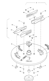
ETB-007802, Tarcze do rozsiewu granicznego TS 10-14
