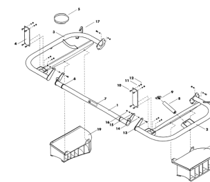
ETB-007830, Składany rurowy pałąk ochronny i trymer
