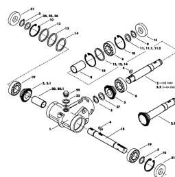
ETB-007808, Przekładnia wejściowa i specjalna przekładnia wejściowa
